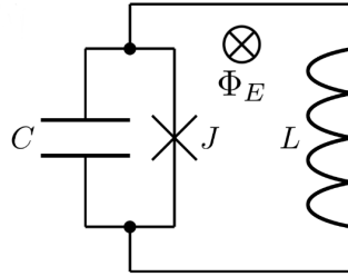
Abbildung 2: Ersatzschaltbild für realen Josephson-Kontakt.
